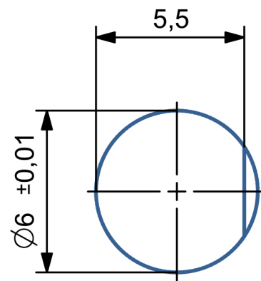
D 字型轴尺寸 比例 5 : 1
