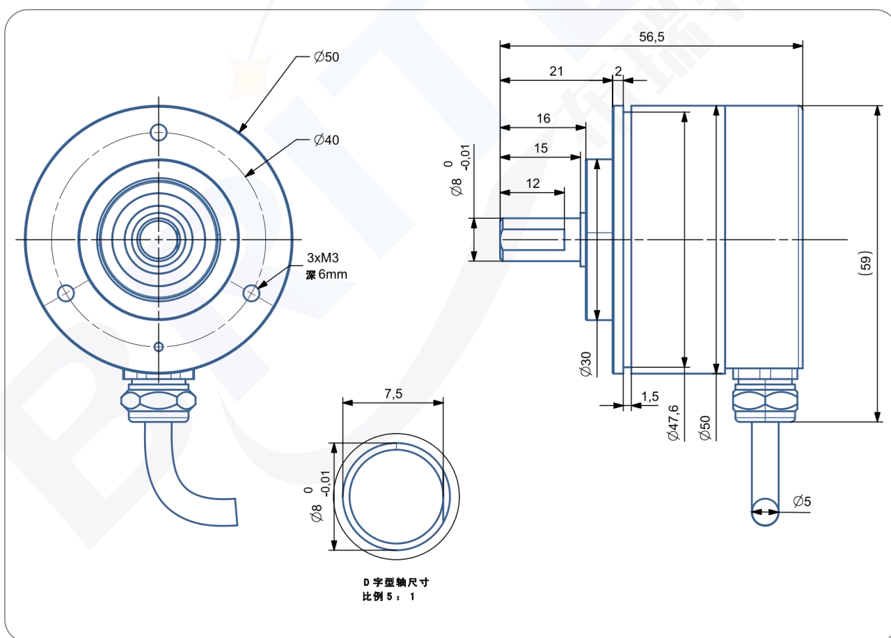
尺寸型号图 12: 输出轴 8mm IP68/防爆
