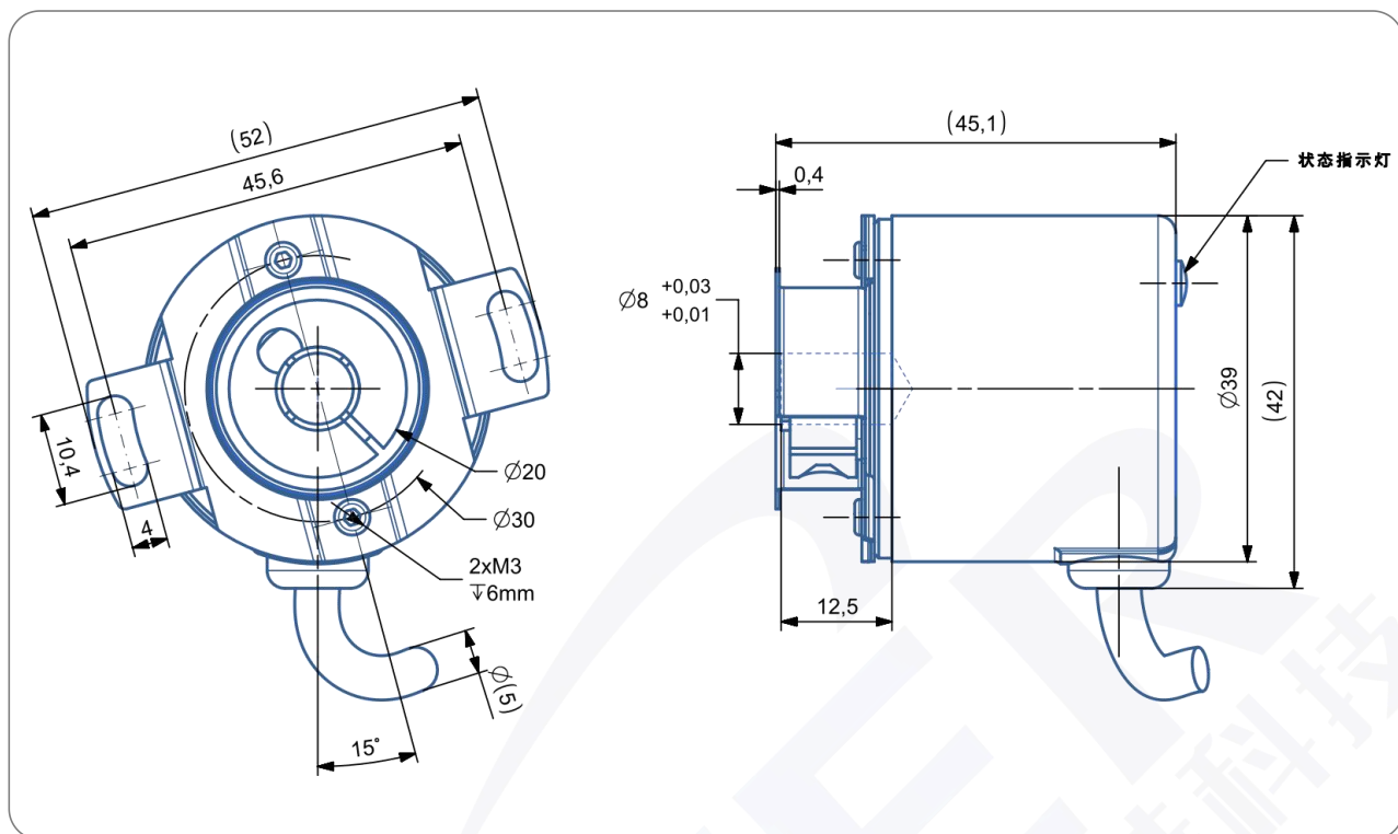
尺寸型号图 3: 抱箍 8mm IP54
