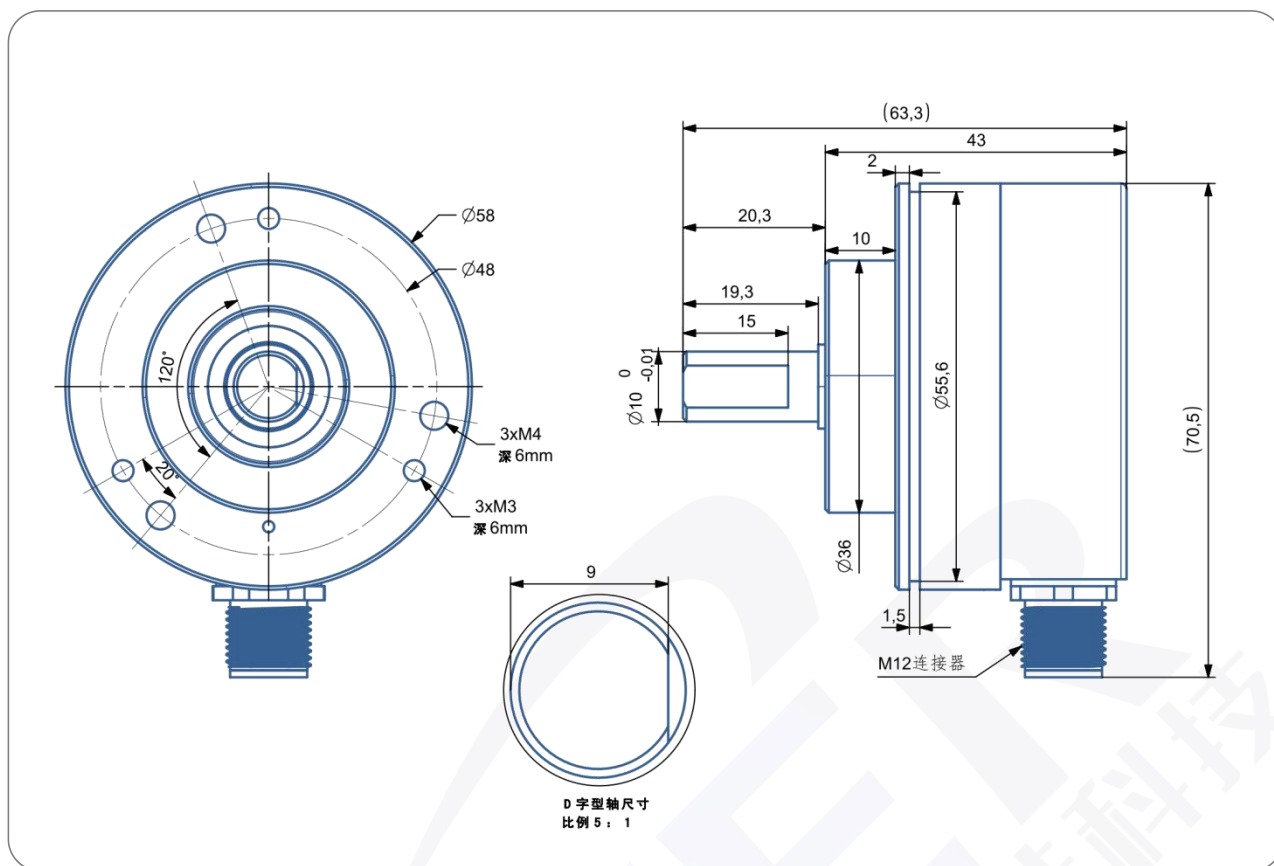
尺寸型号图 14: 输出轴 10mm IP68/防爆
