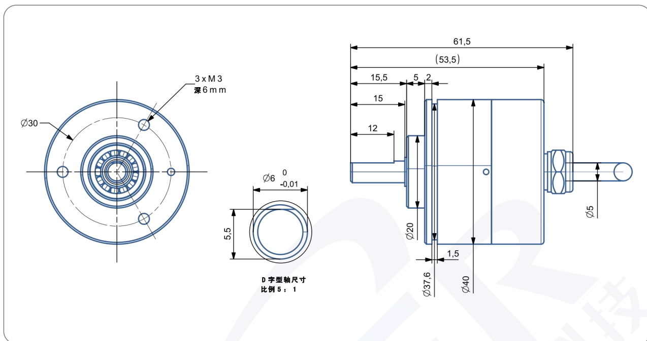
尺寸型号图 9: 输出轴 6mm 尾出 IP68/防爆
