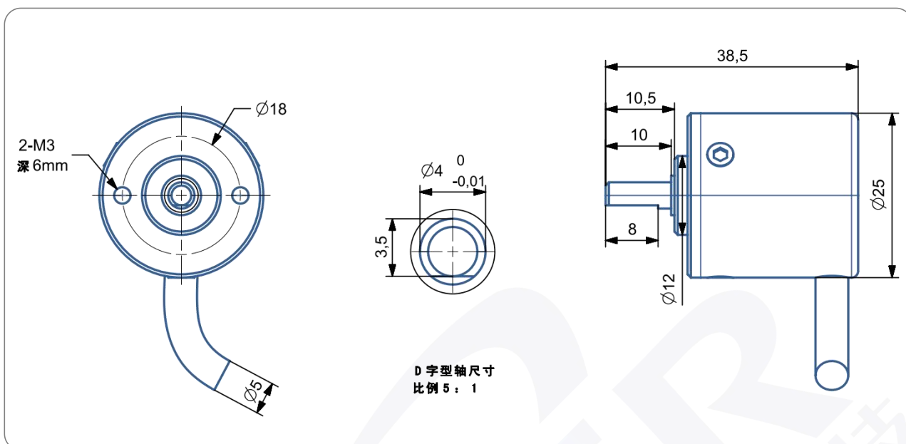
尺寸型号图 7: 输出轴 4mm 侧出 IP54
