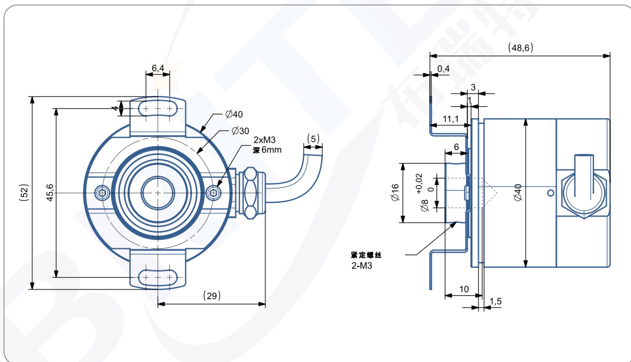
尺寸型号图 10: 输出轴 8mm 盲孔 IP68/防爆
