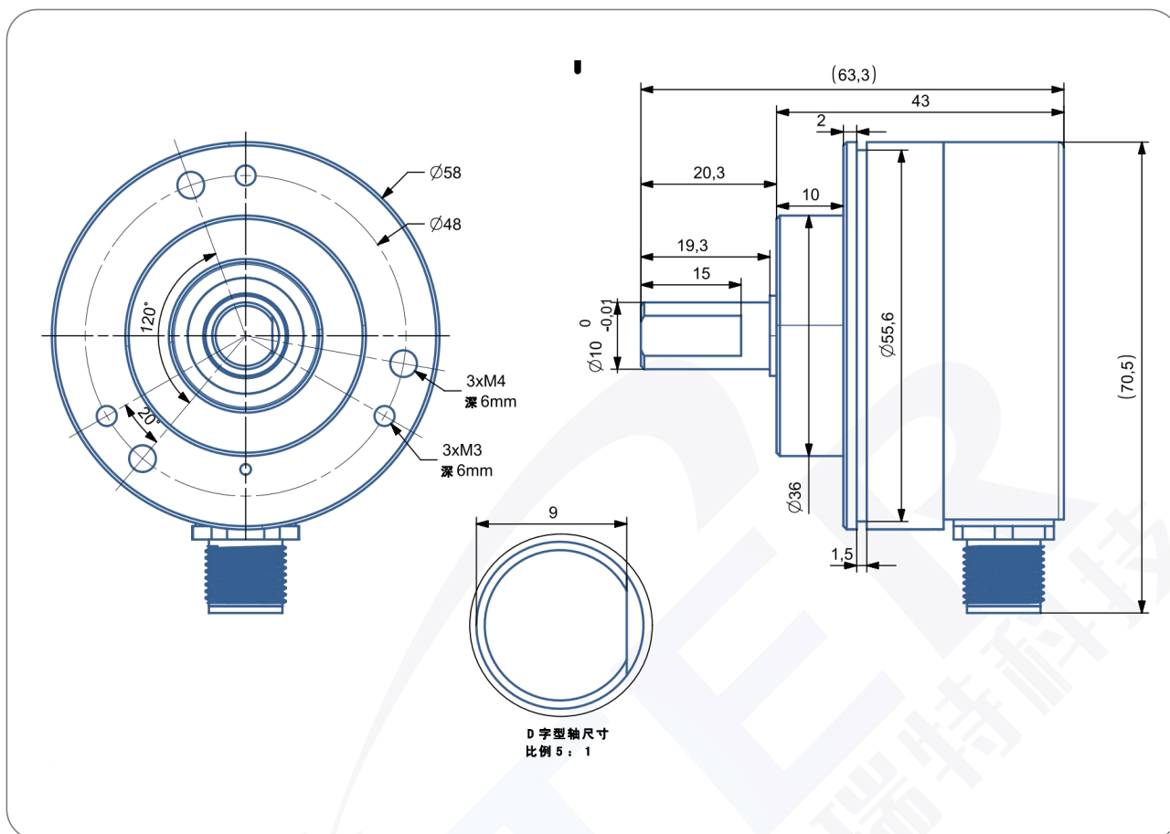
尺寸型号图 12: 输出轴 10mm IP68/防爆
