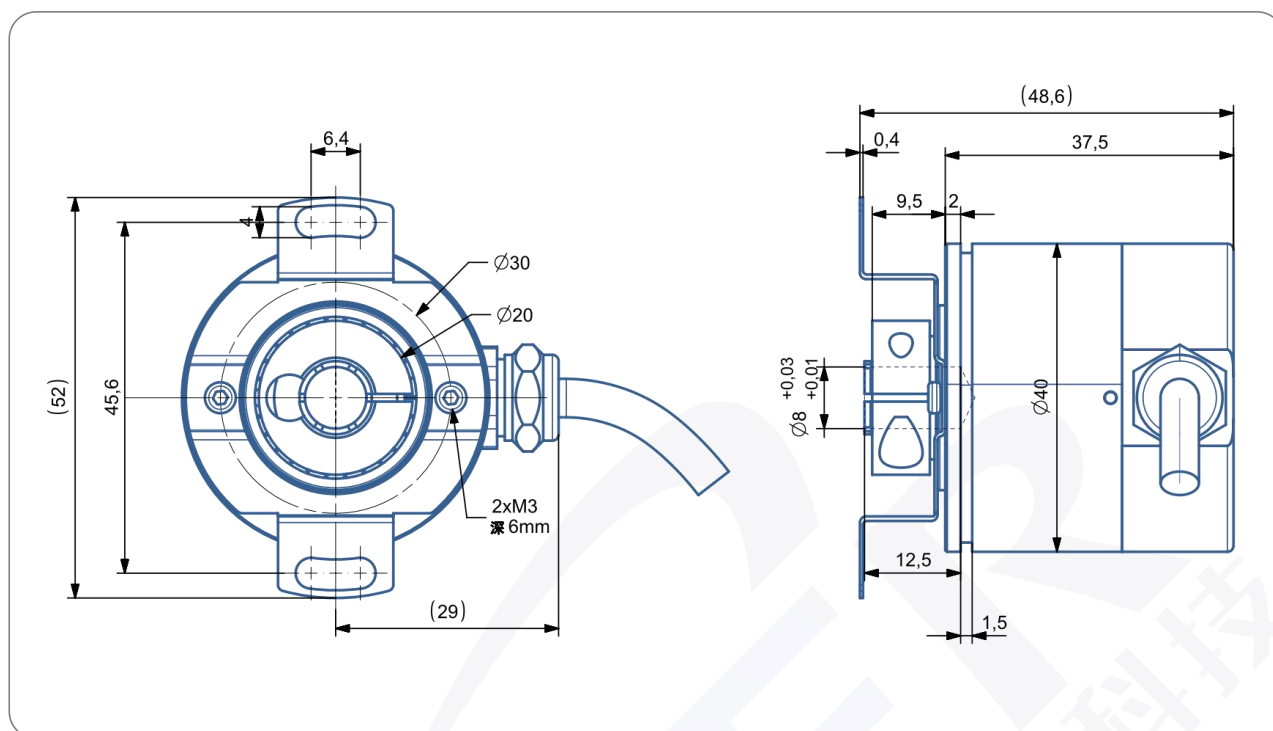
尺寸型号图 11: 抱箍 8mm IP68/防爆
