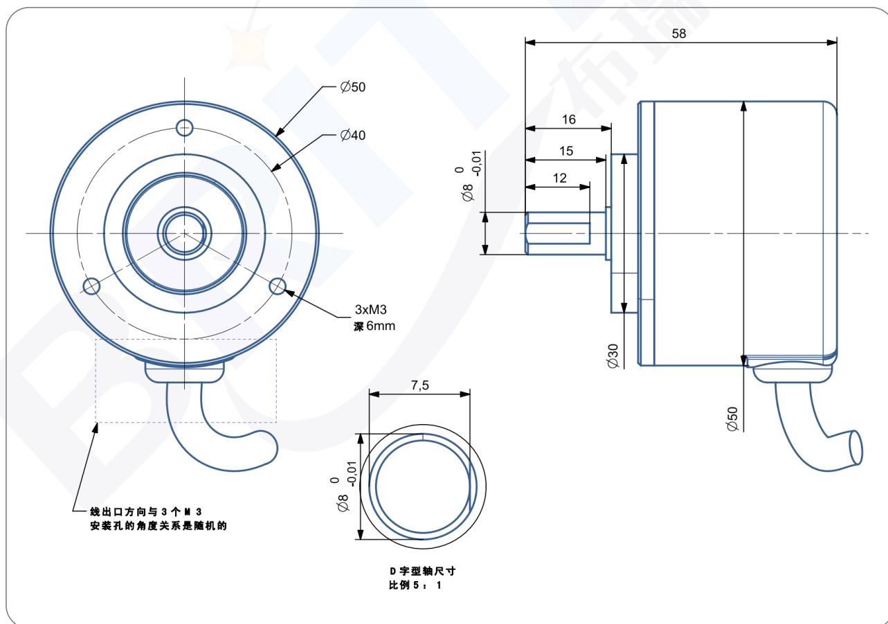
尺寸型号图 3: 抱箍 8mm IP54
