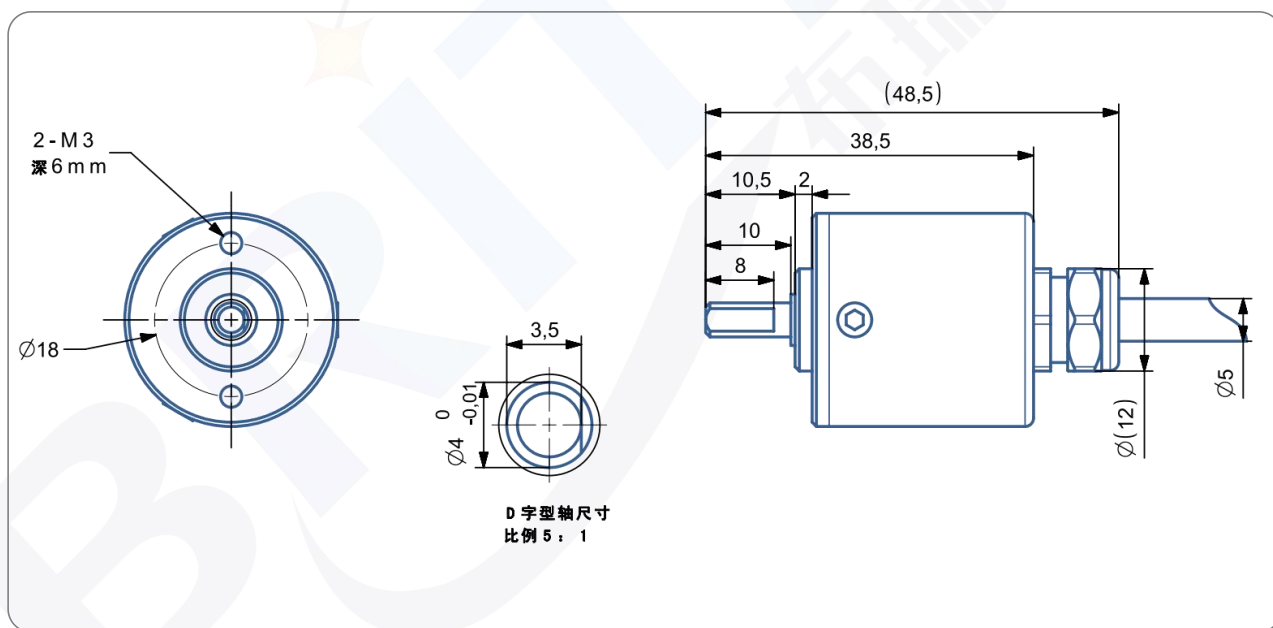
尺寸型号图 6: 输出轴 4mm 尾出 IP54
