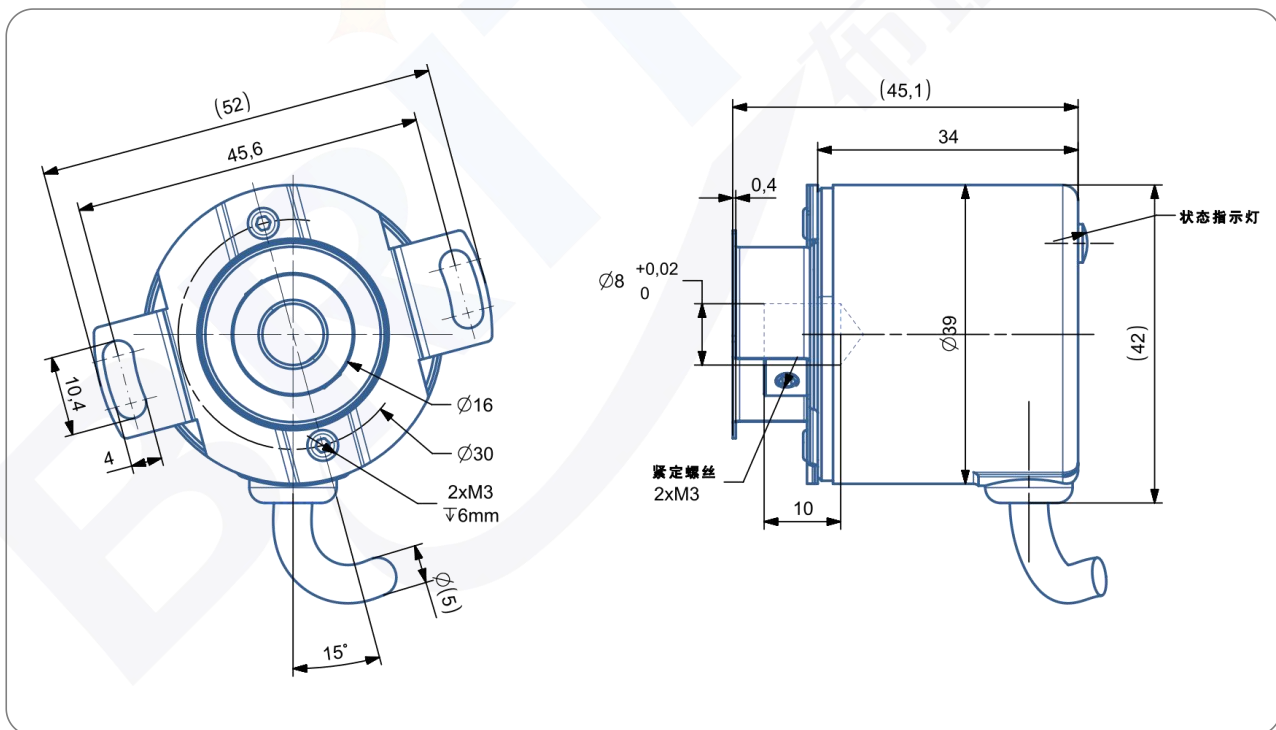
尺寸型号图 2：盲孔 8mm IP54
