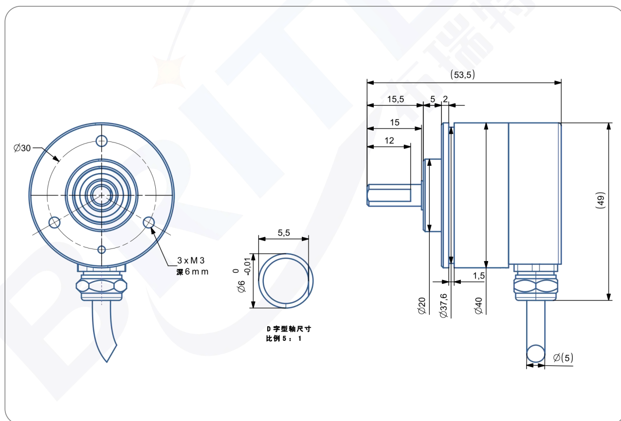
尺寸型号图 8: 输出轴 6mm IP68/防爆
