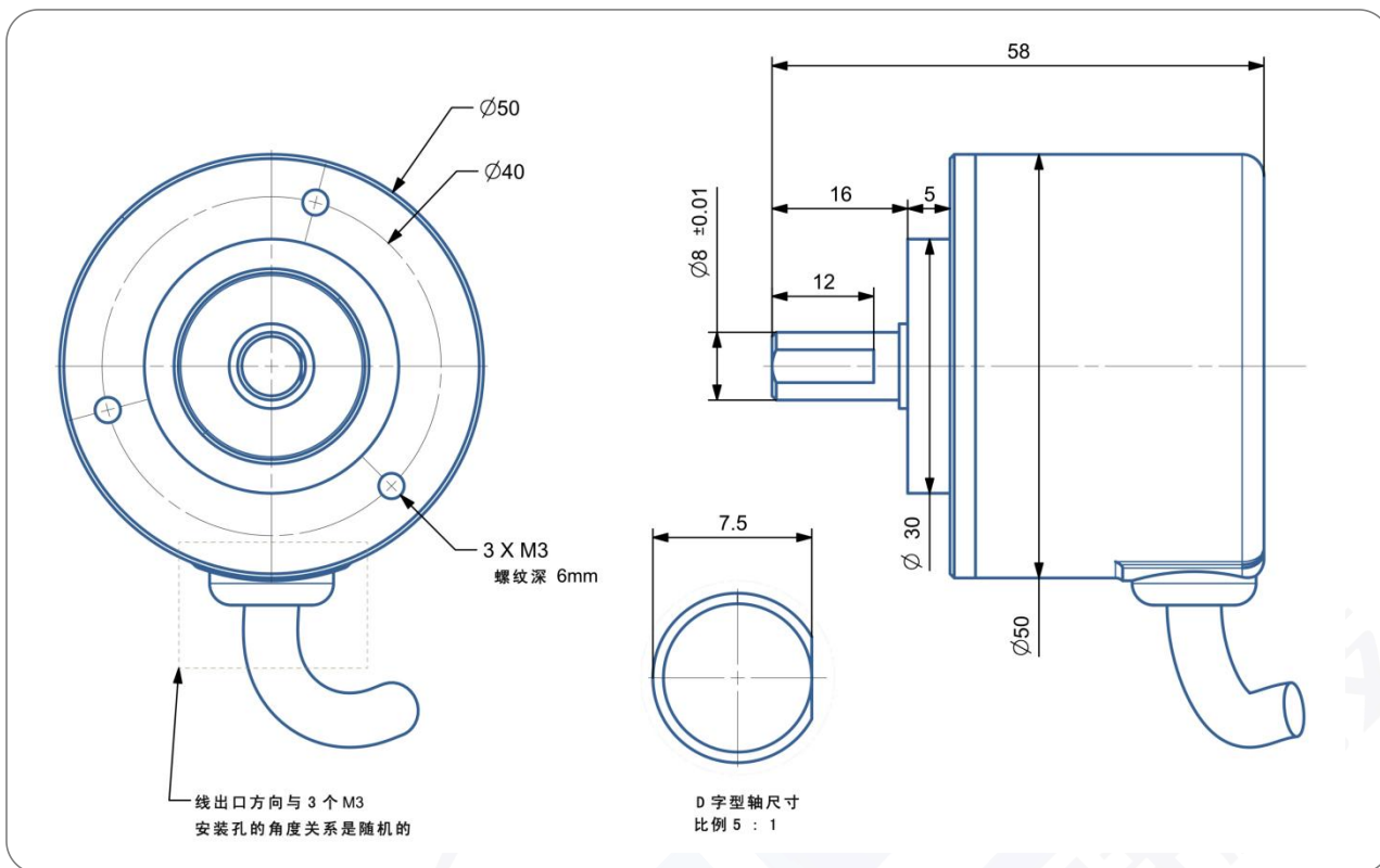
尺寸型号图 5: BRT50 输出轴 10mm IP54
