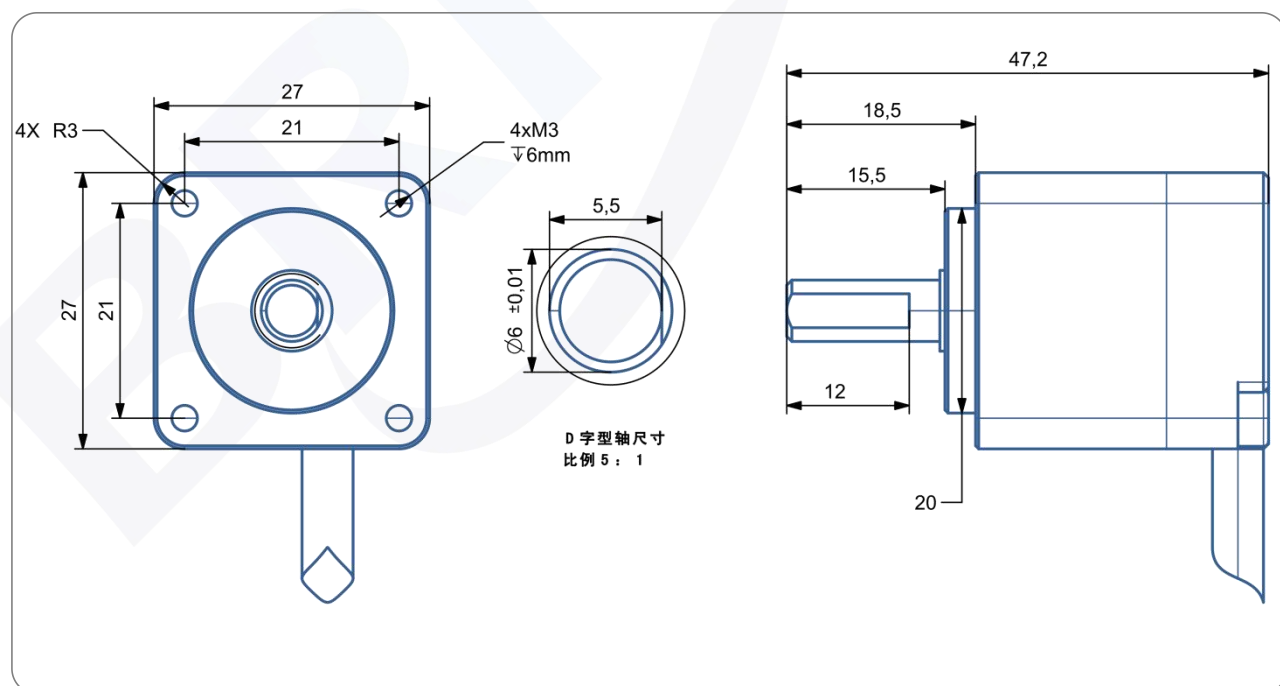
尺寸型号图 13: 输出轴 6mm IP68/防爆
