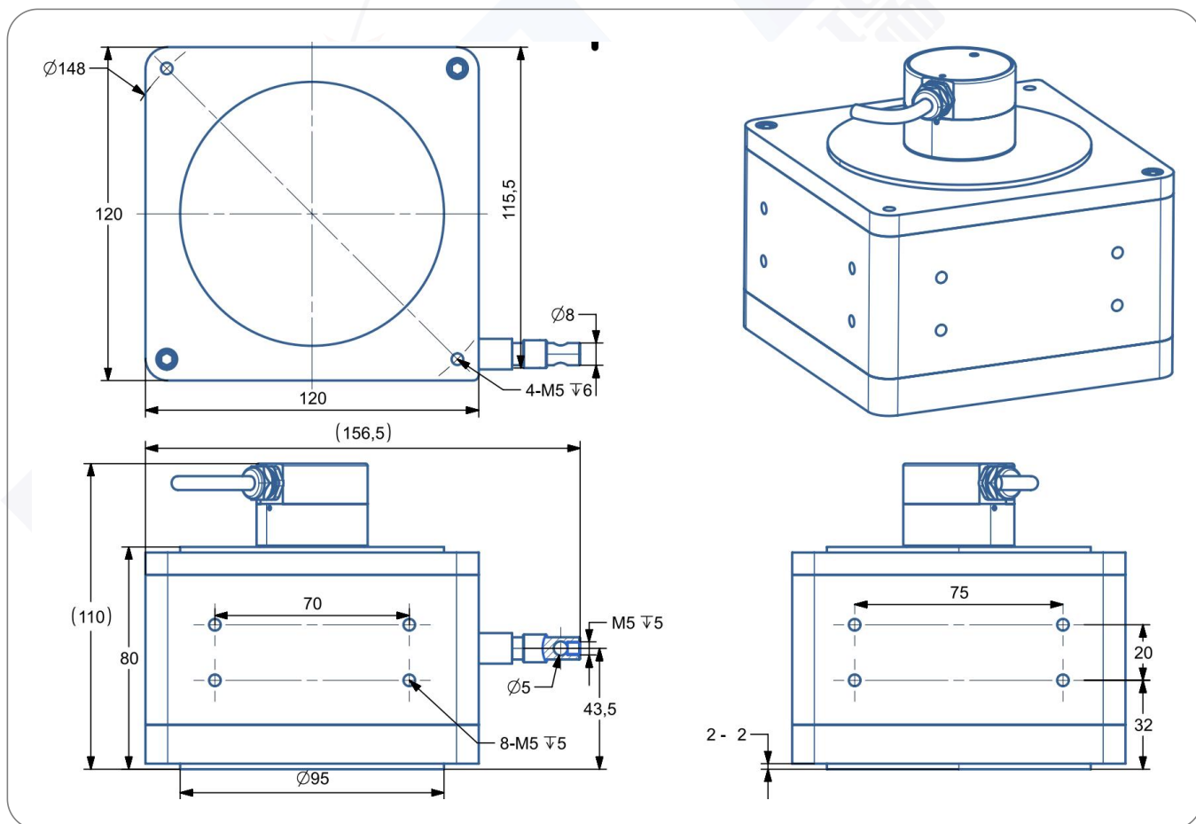
IP68/防爆款 BRT38 系列 8 米/9 米/10 米拉绳位移传感器安装尺寸图
