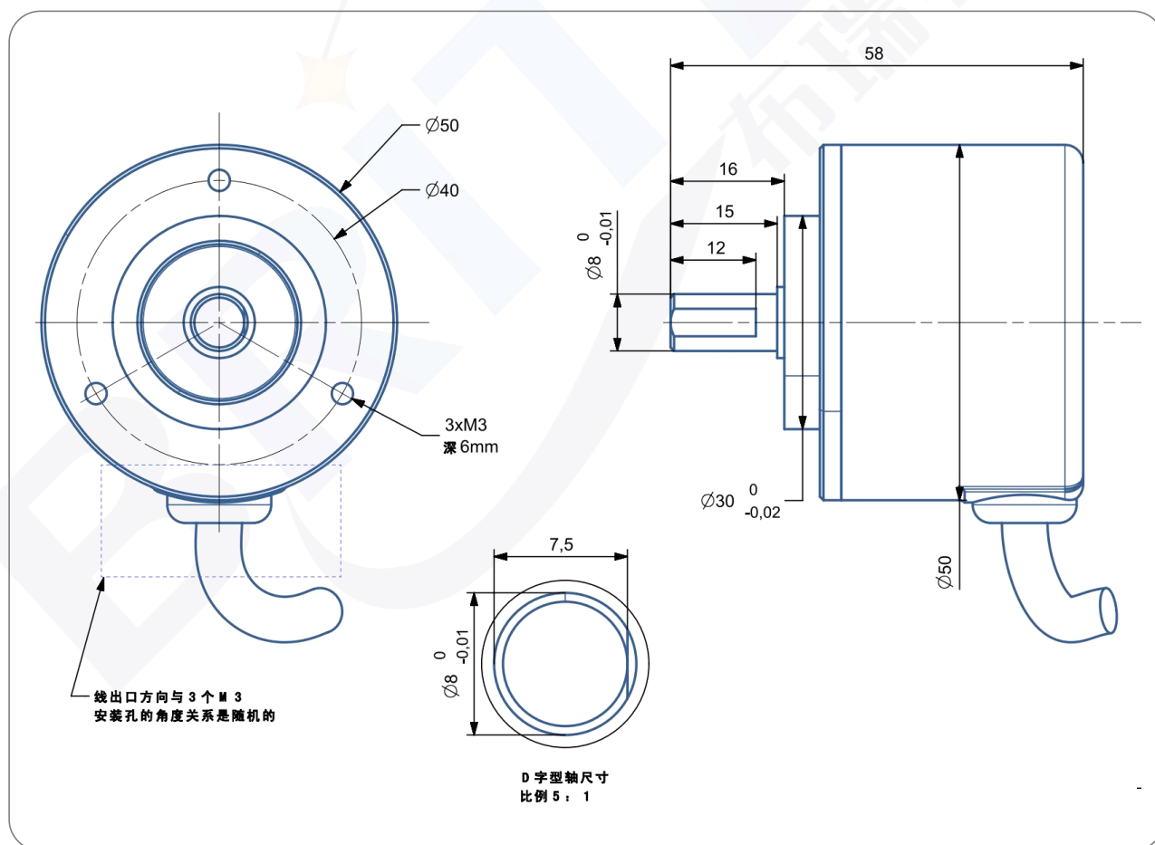
尺寸型号图 4: 输出轴 8mm IP54
