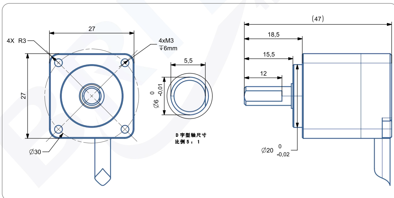
尺寸型号图 8： 输出轴 6mm 轴 IP68/防爆
